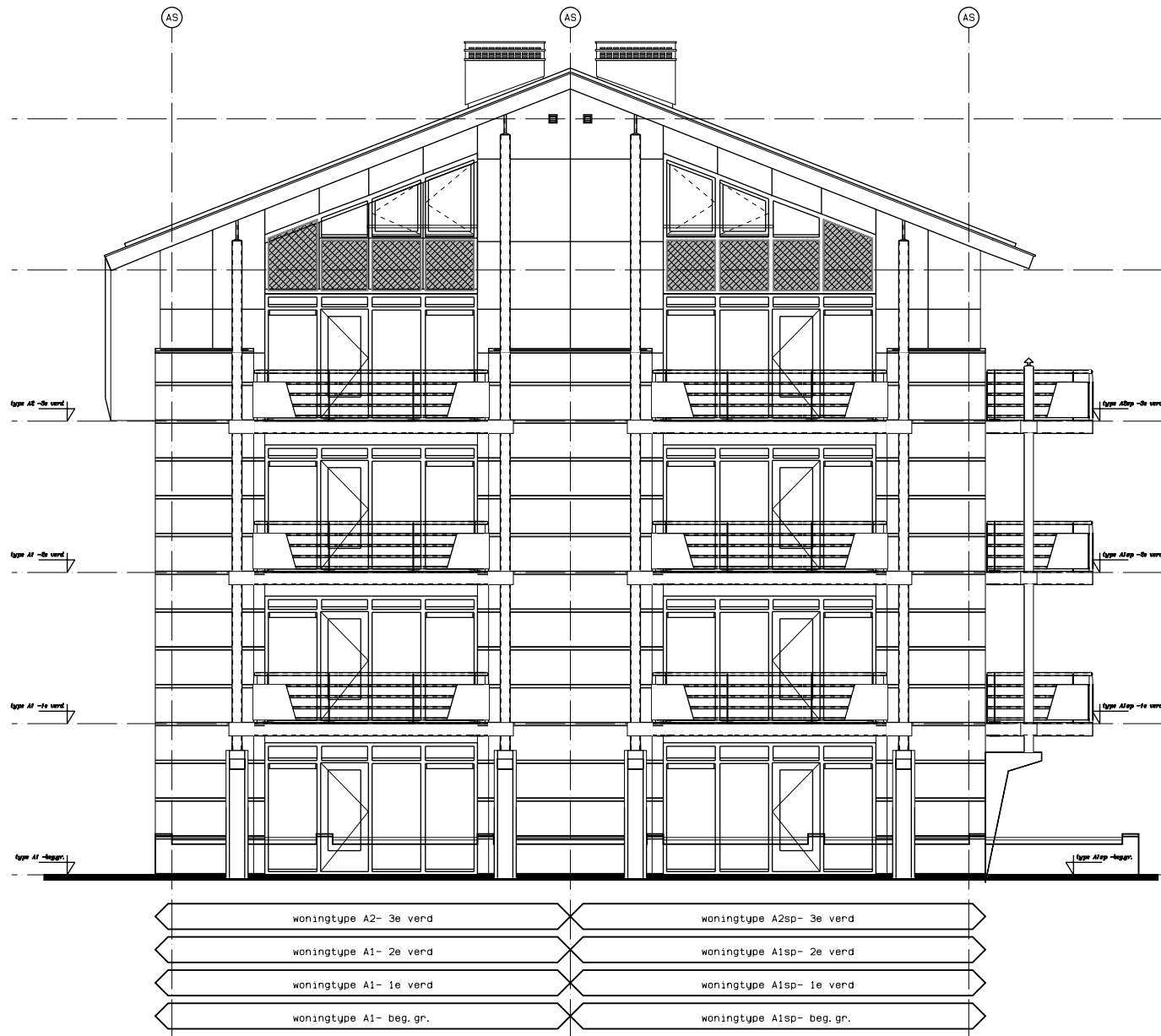
Zuidgevel
